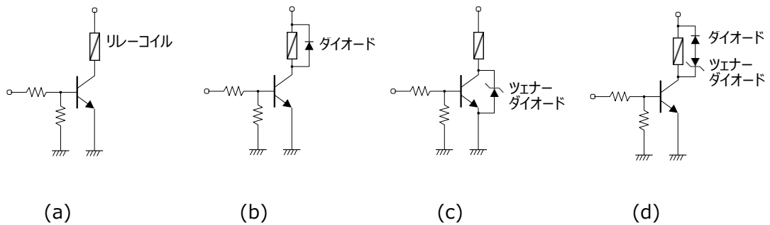
図8 駆動回路
