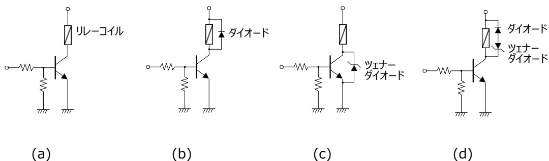
図8 駆動回路
