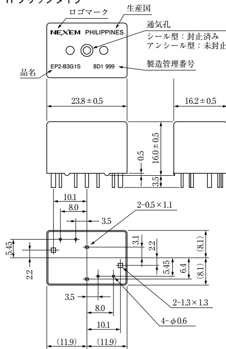
“H”ブリッジタイプ
