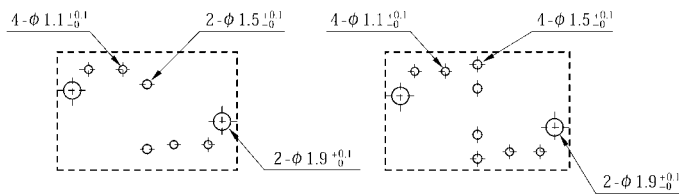
〔“H”ブリッジタイプ〕
