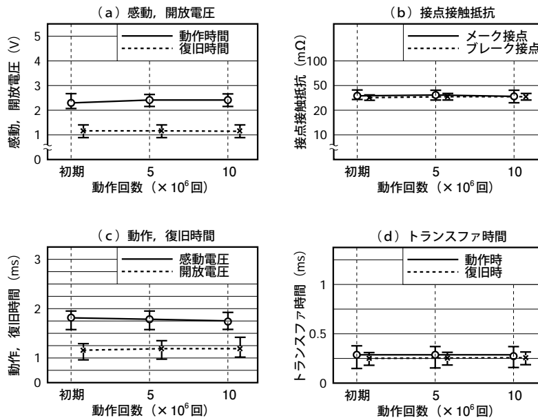
図5-10 無負荷試験B
