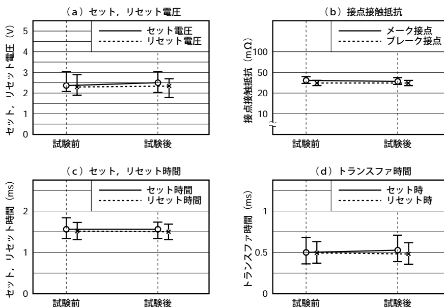
図5-5 (2) 振動
