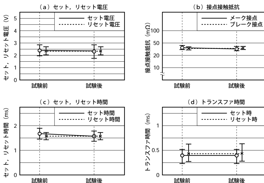
図5-4 (2) 熱衝撃
