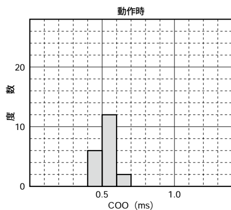
図4-4D 時間特性
