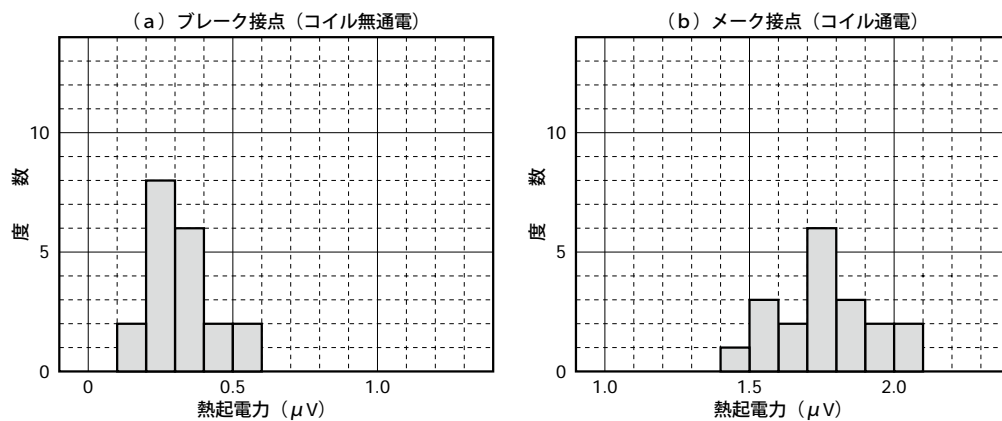
図4-7 熱起電力
