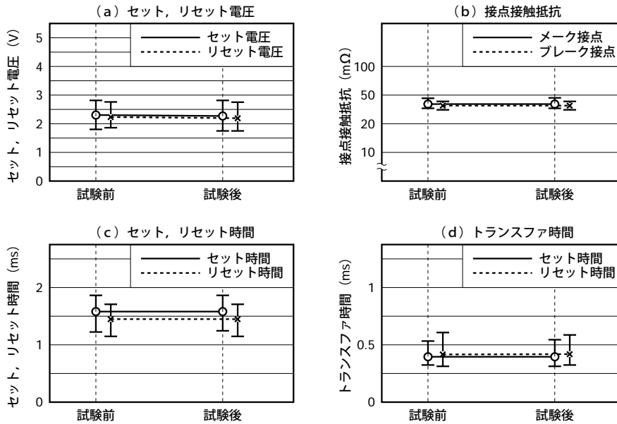
図5-2 (2) 低温放置
