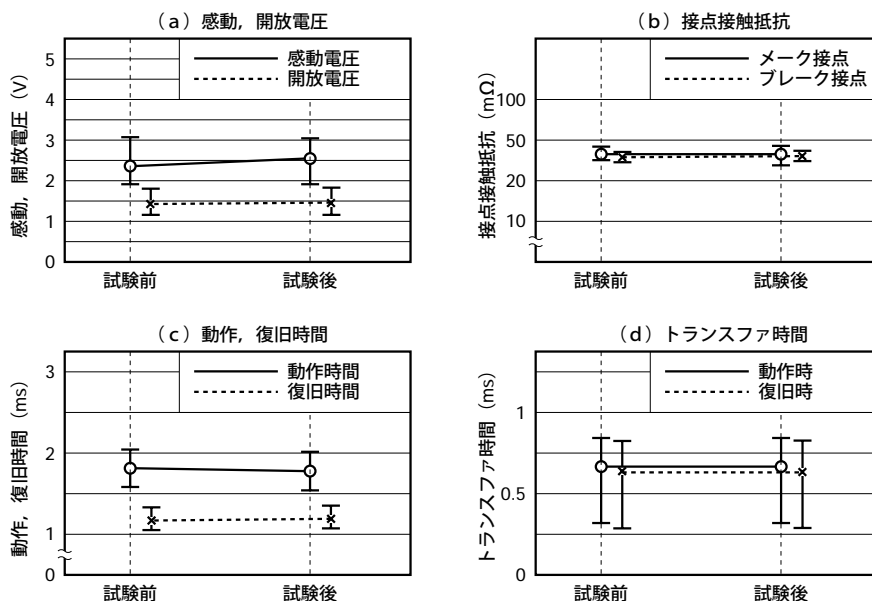
図5-5 (1) 振動
