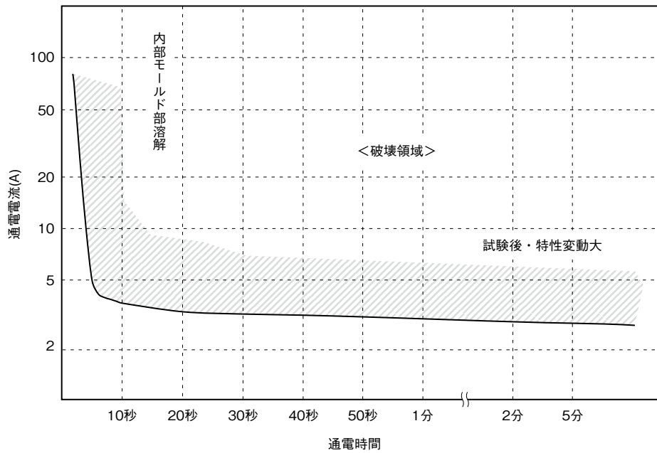
図3-12 通電耐量
