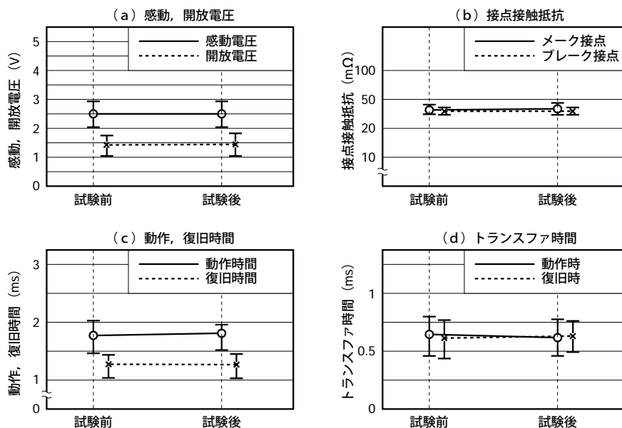
図5-6 (1) 衝撃
