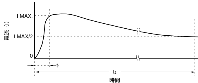
図3-11 電流サージ耐量
