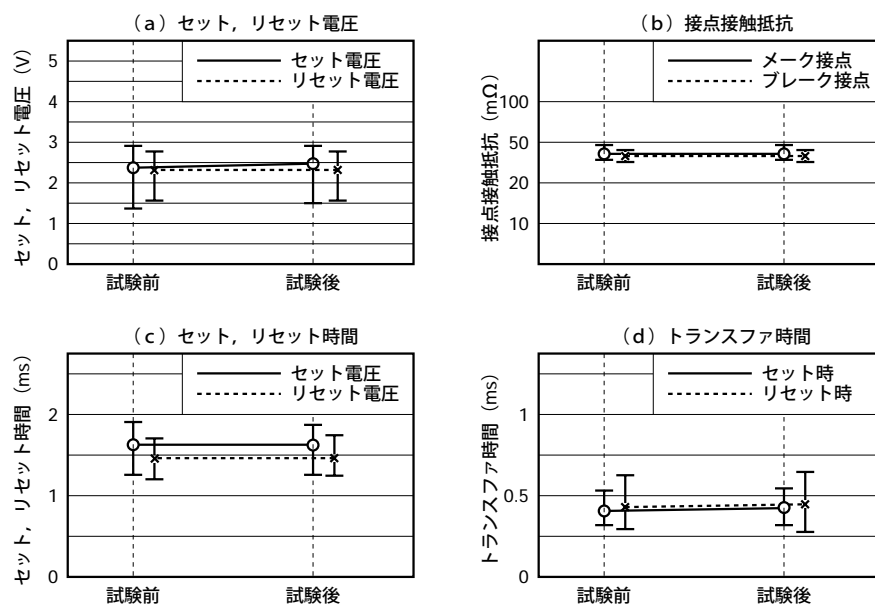
図5-3 (2) 温湿度サイクル
