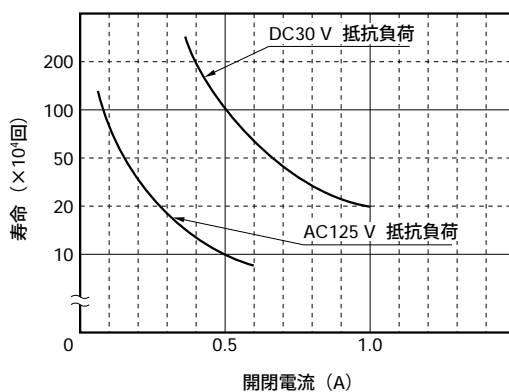
図3-2 寿命曲線
