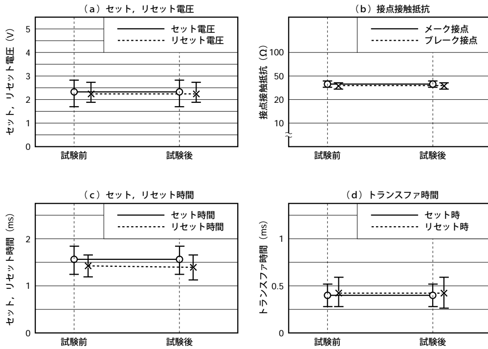
図5-1 (2) 高温放置
