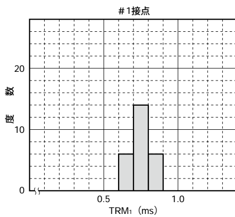
図4-4B 時間特性
