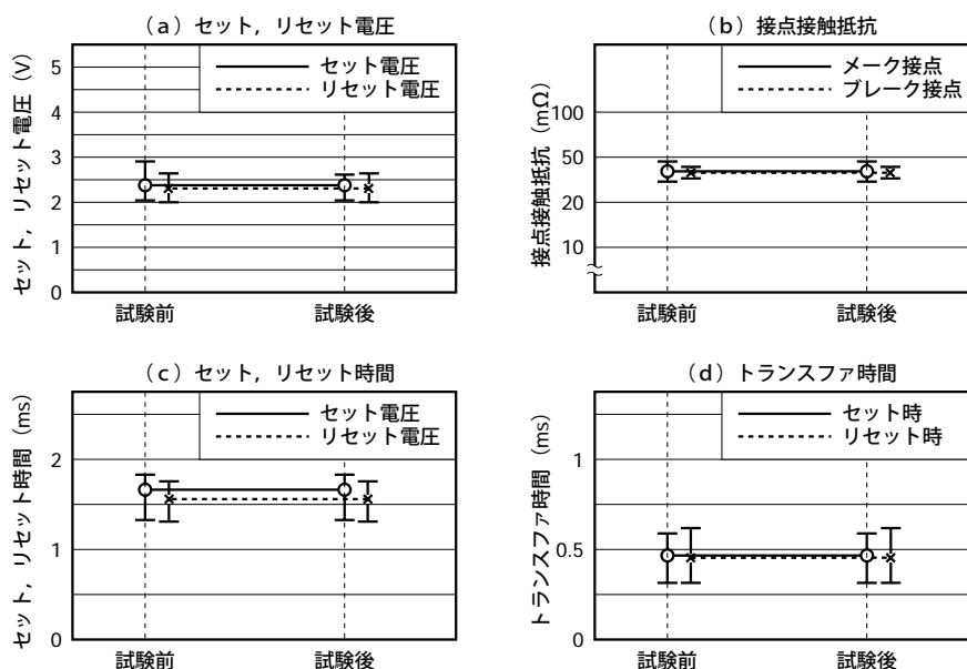
図5-8 (2) 端子強度
