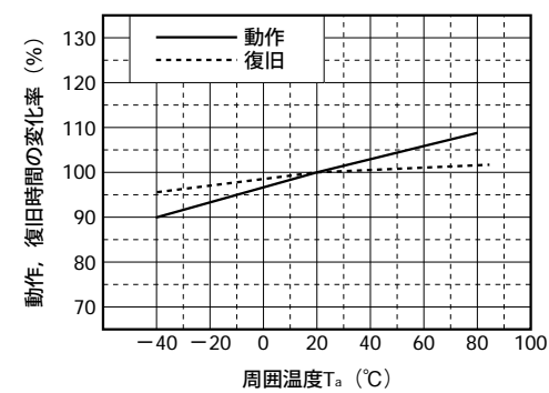
図3-7 温度特性
