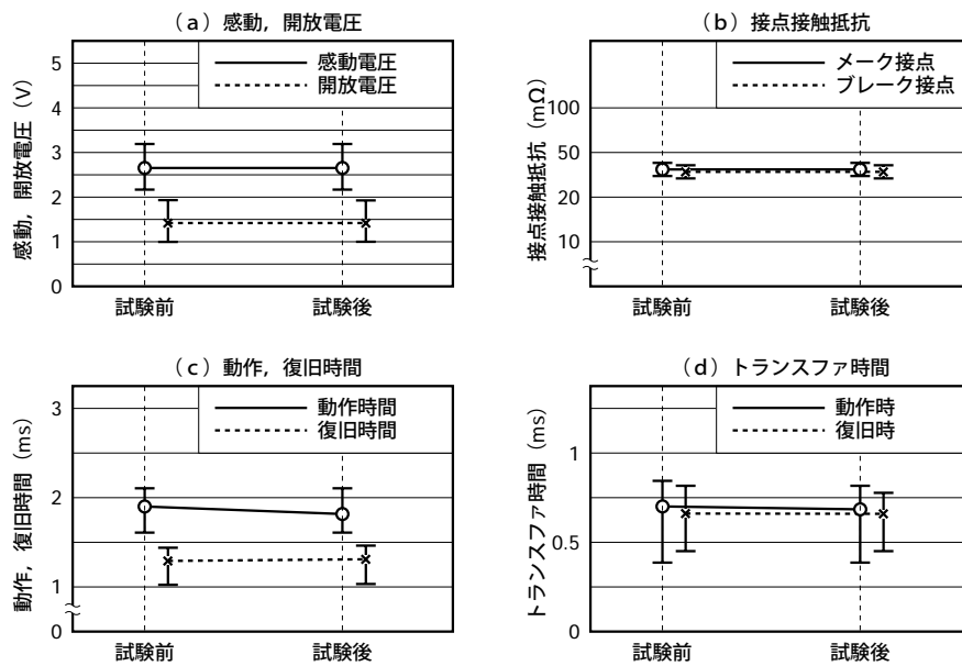
図5-3 (1) 温湿度サイクル
