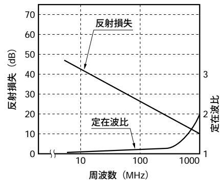
図3-9 高周波特性
