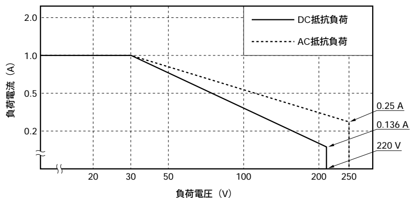
図3-1 開閉容量
