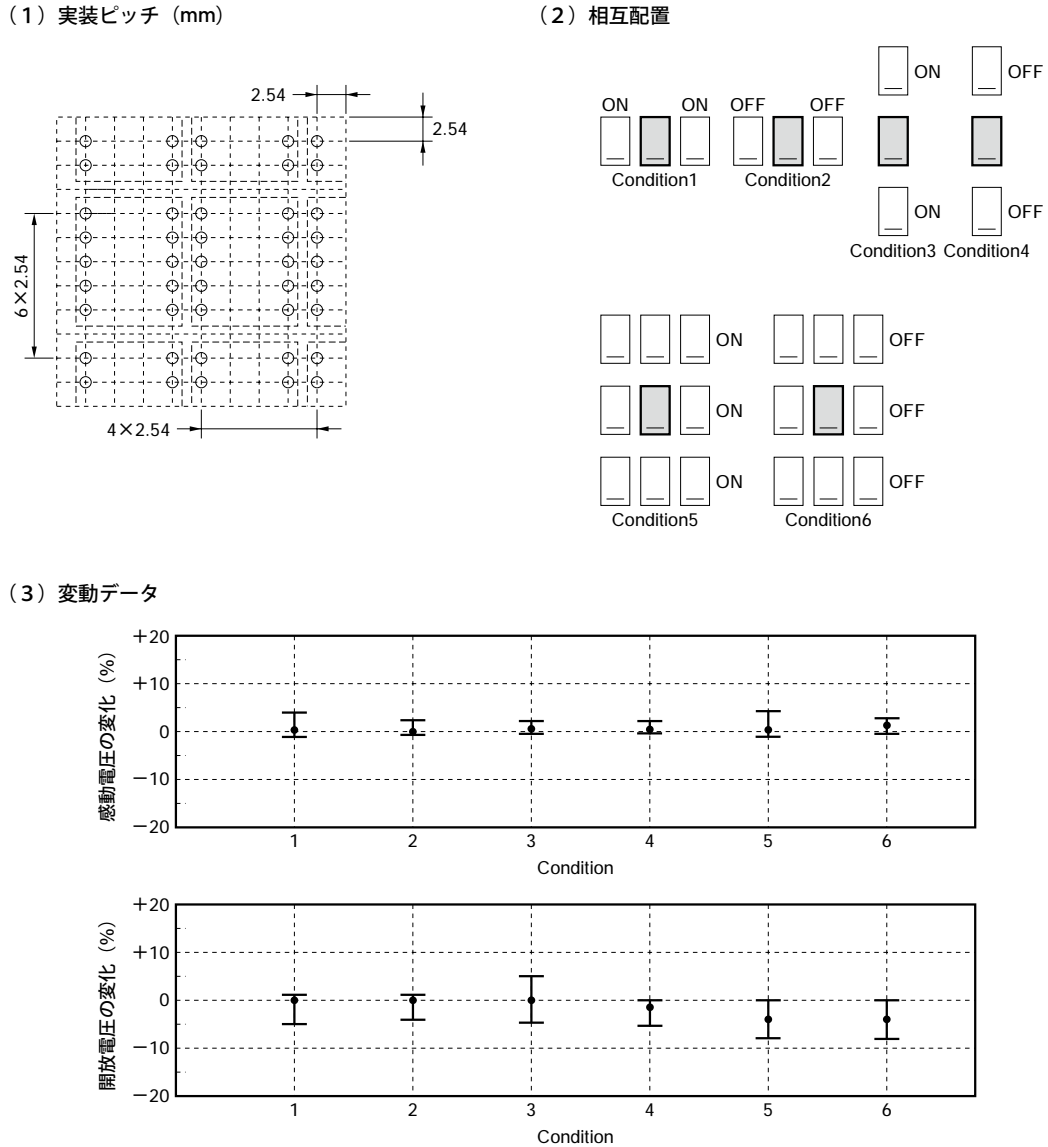
図3-8 磁気干渉
