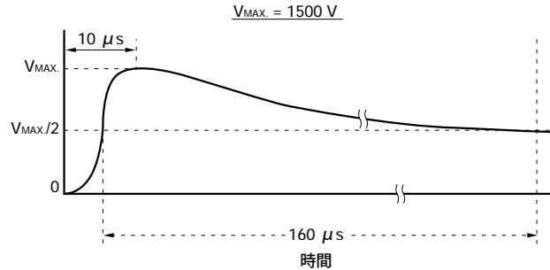
図3-10 電圧サージ耐量
