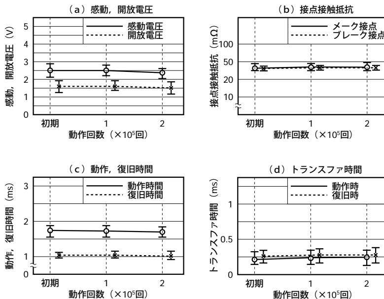
図5-17 抵抗負荷試験F
