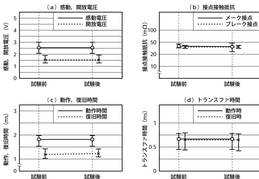
図5-4 (1) 熱衝撃
