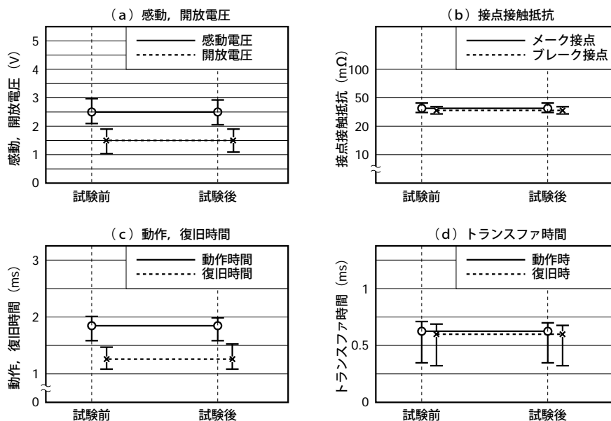
図5-8 (1) 端子強度
