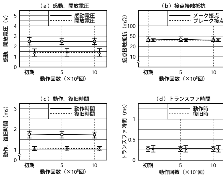
図5-14 抵抗負荷試験D
