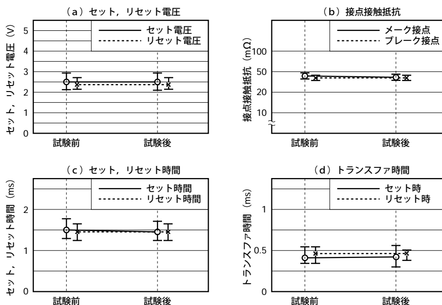
図5-7 (2) はんだ耐熱
