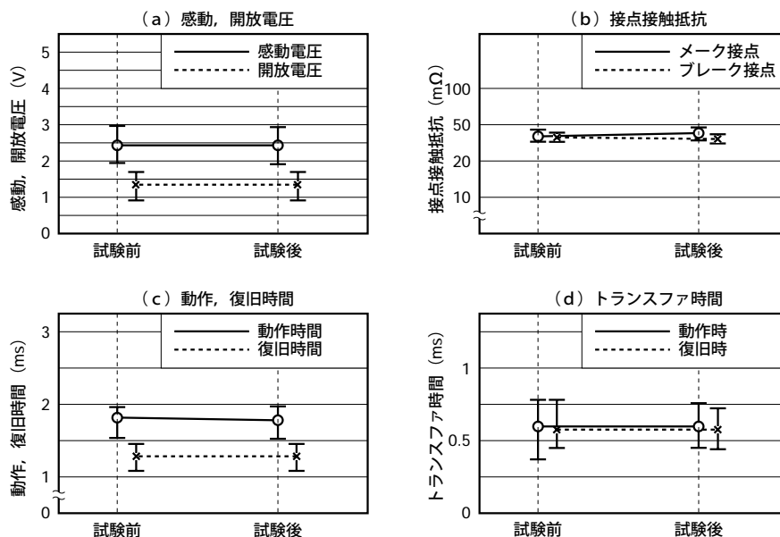
図5-7 (1) はんだ耐熱
