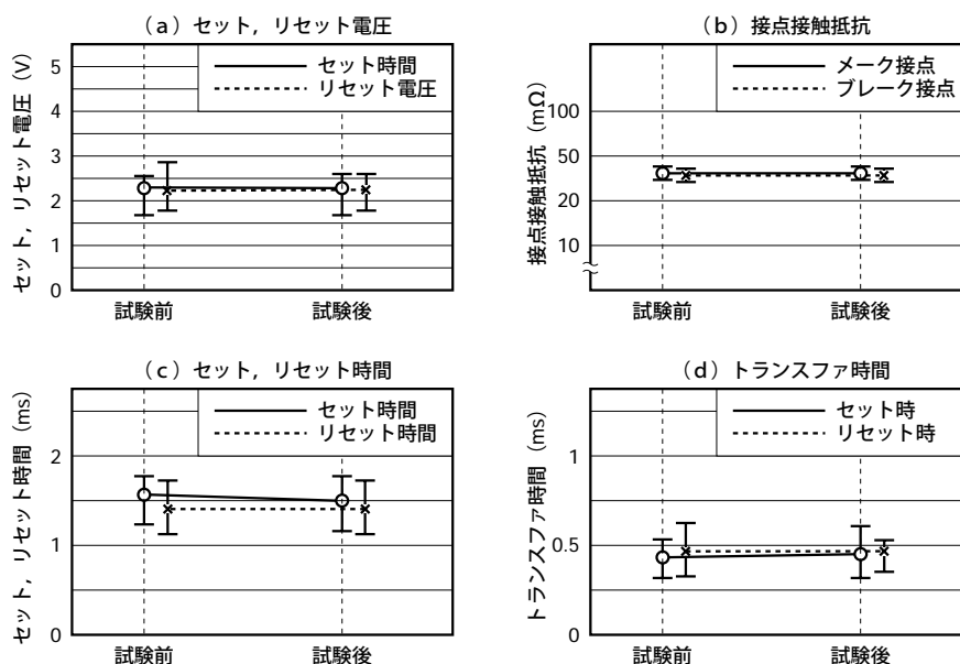
図5-6 (2) 衝撃
