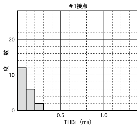
図4-4C 時間特性
