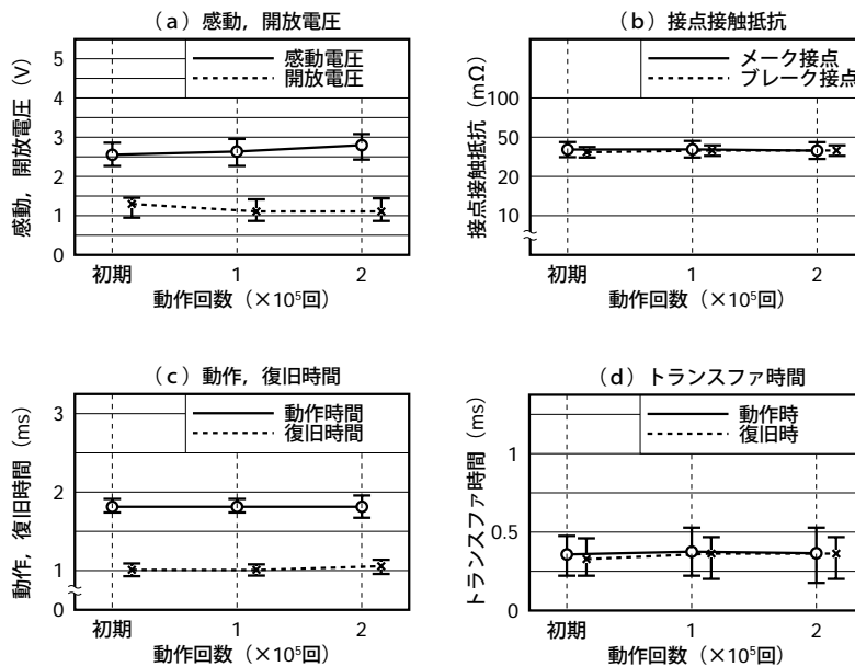
図5-19 抵抗負荷試験H
