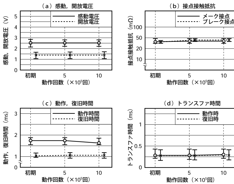
図5-16 誘導負荷試験
