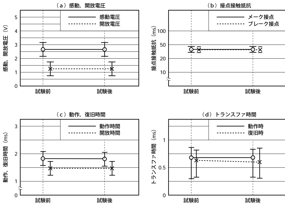
図5-1 (1) 高温放置
