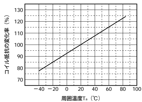
図3-7 温度特性
