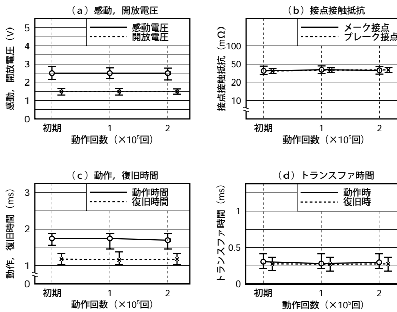
図5-18 抵抗負荷試験G
