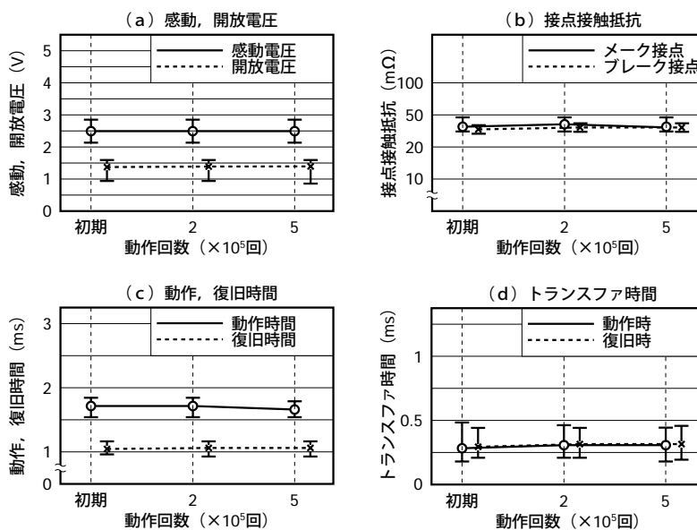
図5-13 抵抗負荷試験C
