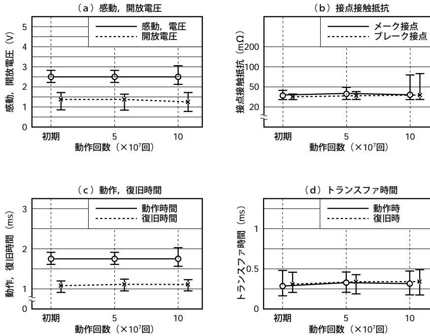
図5-9 無負荷試験A
