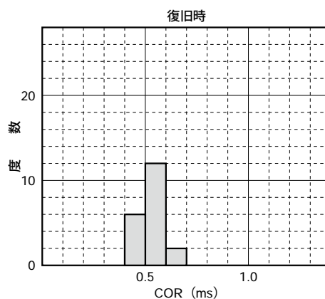
図4-4D 時間特性
