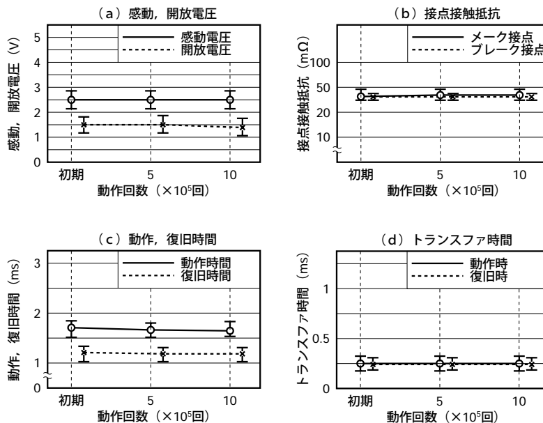
図5-15 抵抗負荷試験E
