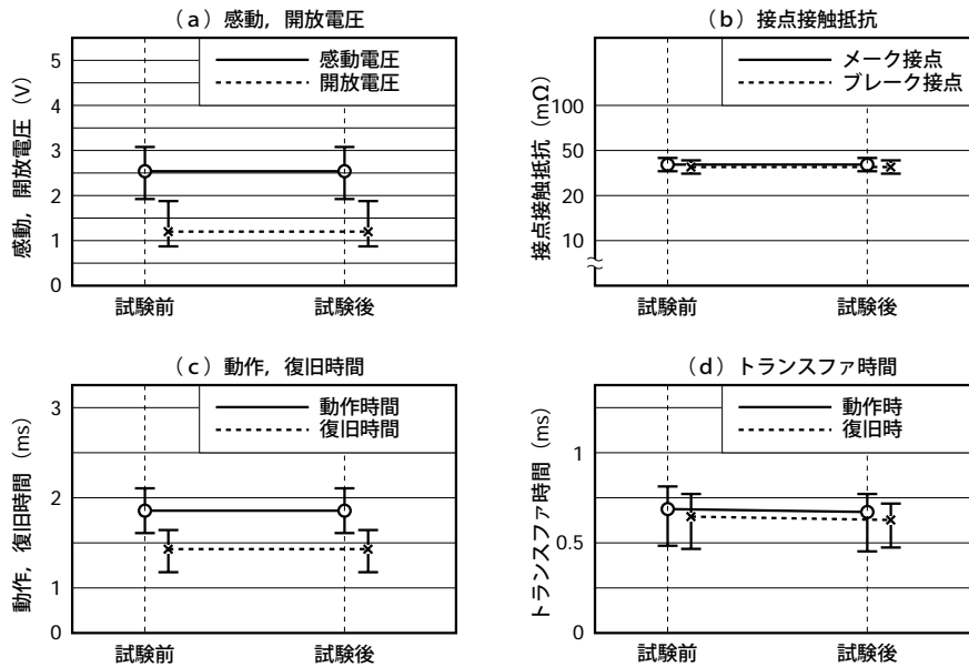
図5-2 (1) 低温放置
