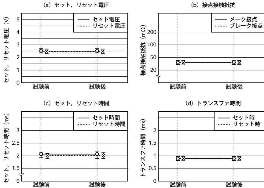
図5.3 (2) 温湿度サイクル
