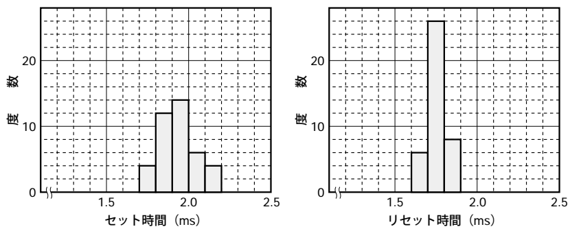
図4.2 動作, 復旧時間
