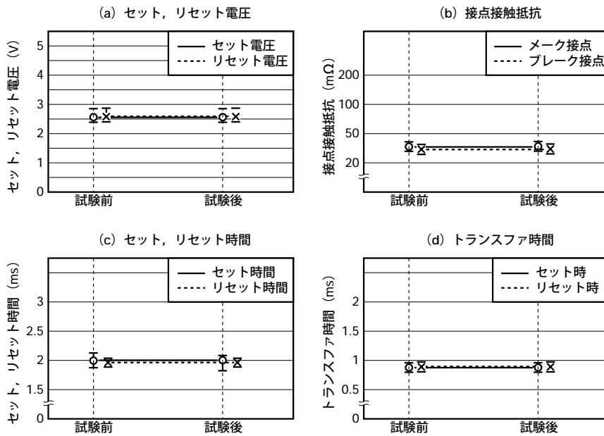
図5.3 (4) 温湿度サイクル
