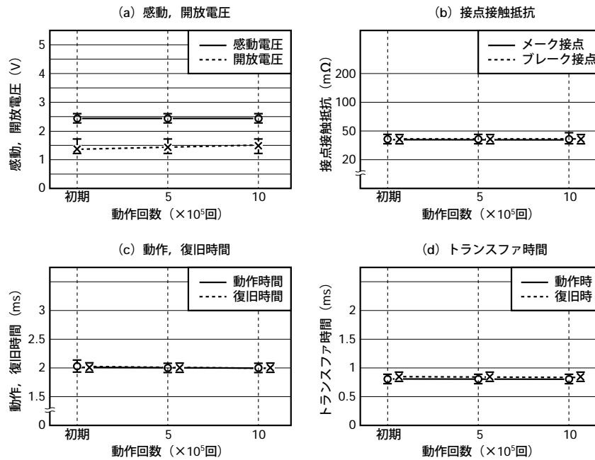
図5.15 抵抗負荷試験D
