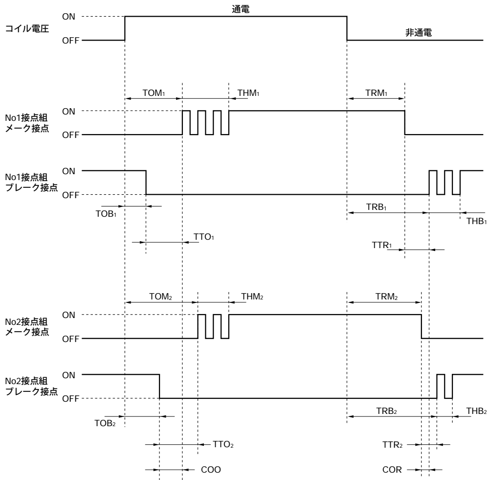
図4.4A コイル、接点のタイミングチャート
