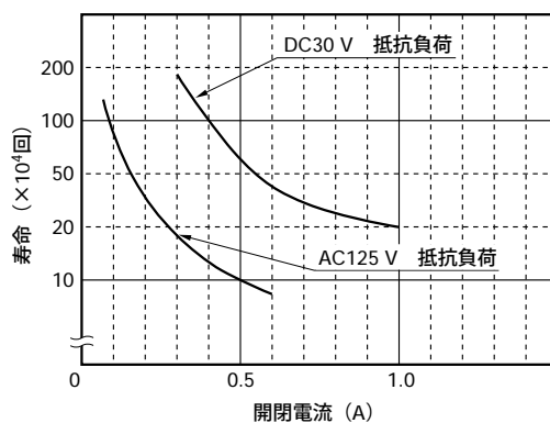
図3. 2 寿命曲線
