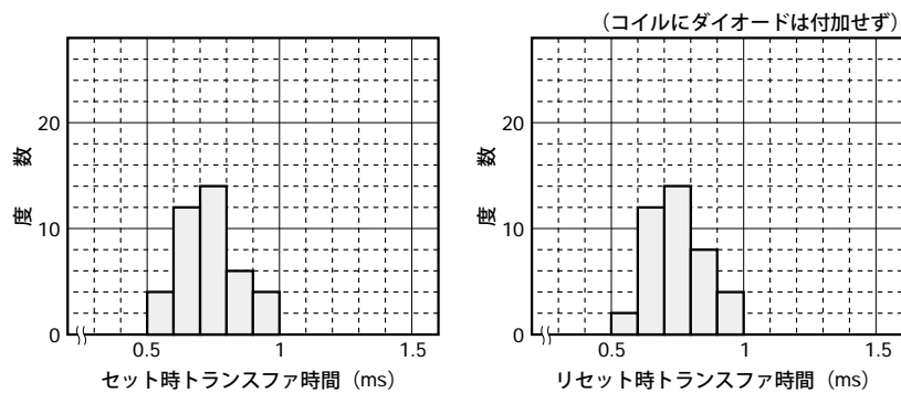
図4.3 トランスファ時間
