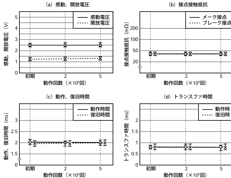
図5.14 抵抗負荷試験C
