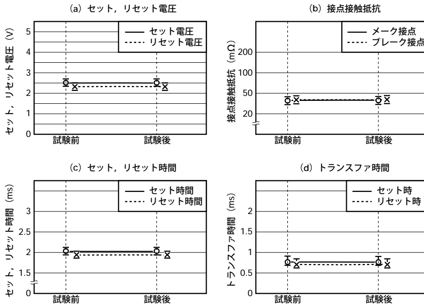
図5.1 (4) 高温放置
