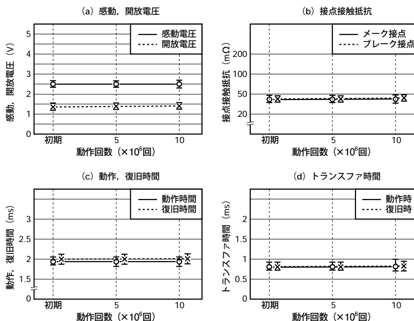
図5.11 無負荷試験B
