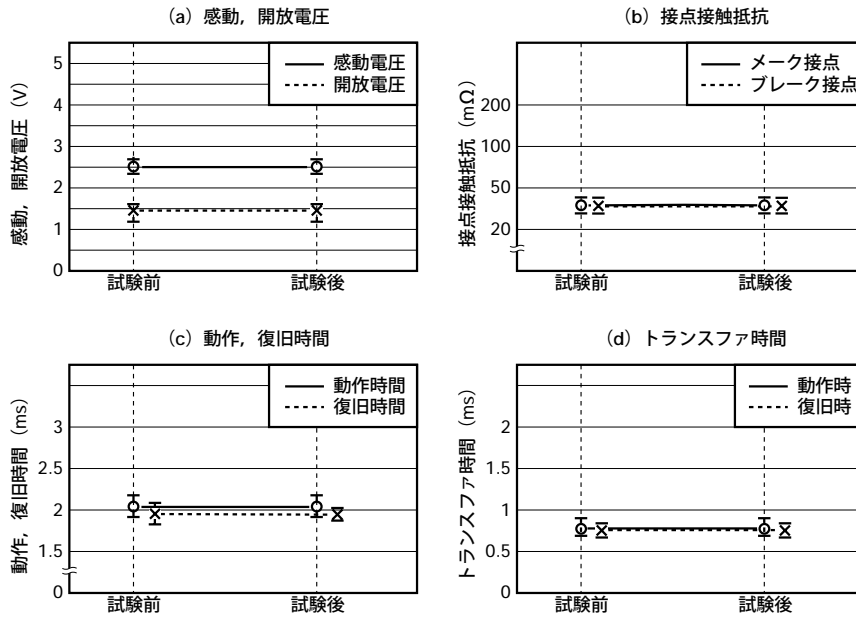
図5.2 (3) 低温放置
