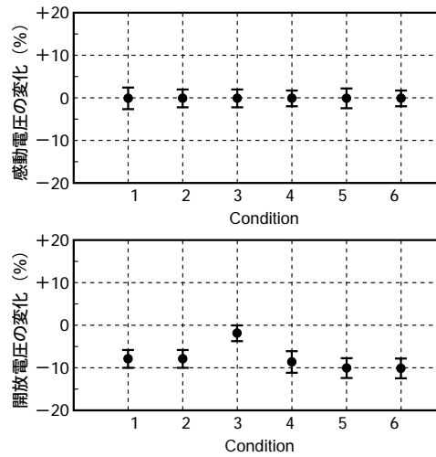
図3.8 磁気干渉
