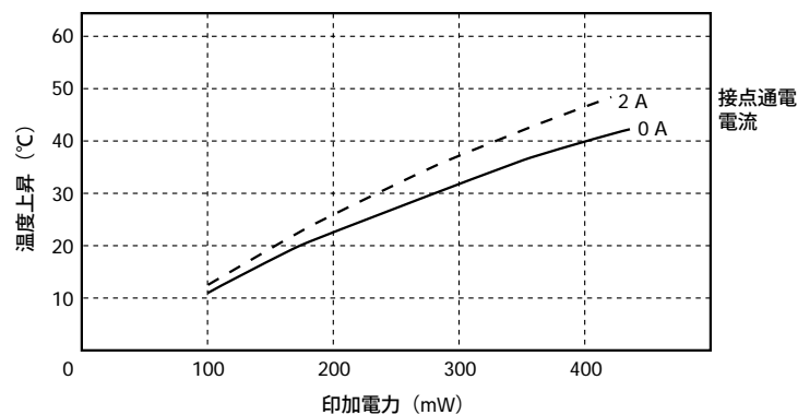
図3.4 コイル温度上昇
