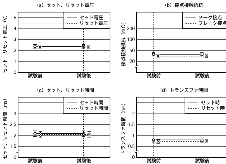
図5.4 (4) 熱衝撃
