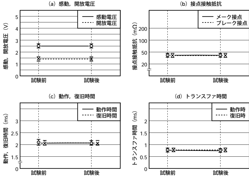
図5.3 (1) 温湿度サイクル
