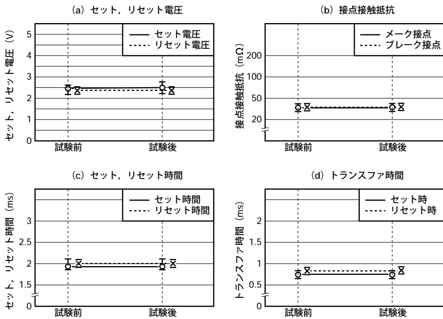
図5.5 (4) 振動
