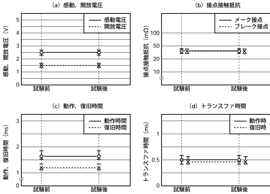
図5.8 (2) リフローはんだ耐熱
