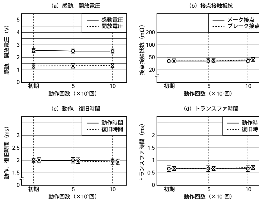
図5.17 誘導負荷試験
