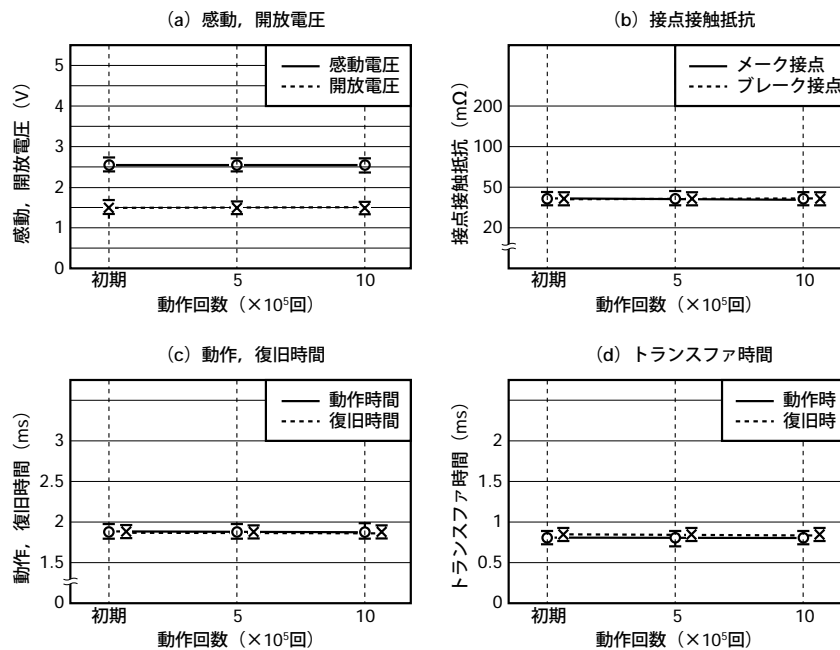
図5.16 抵抗負荷試験E
