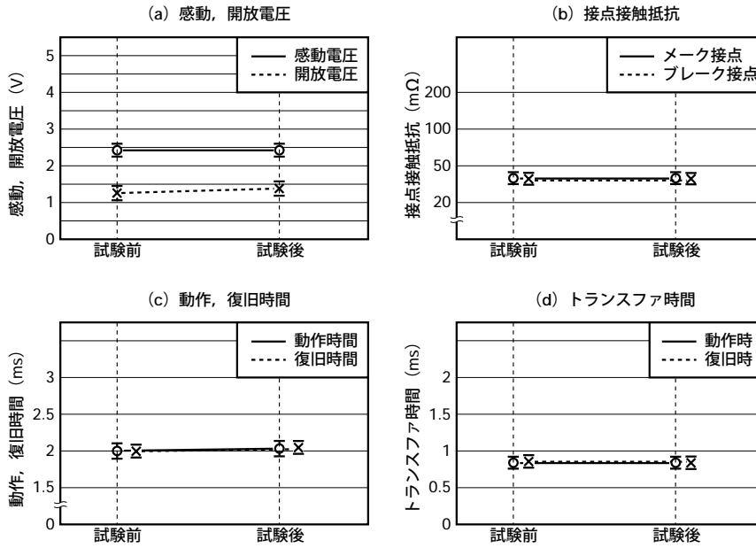
図5.9 (1) 端子強度
