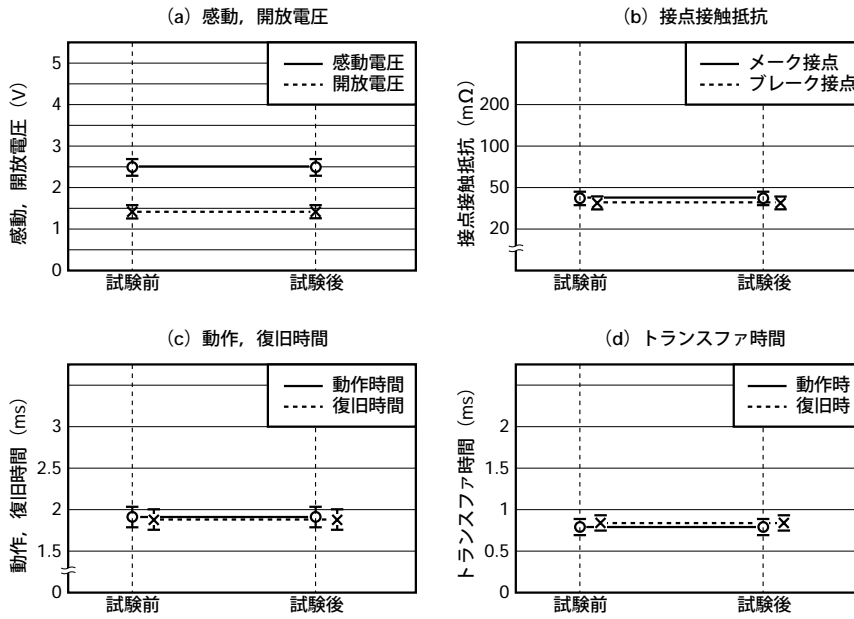
図5.4 (3) 熱衝撃
