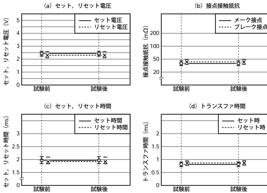
図5.2 (4) 低温放置
