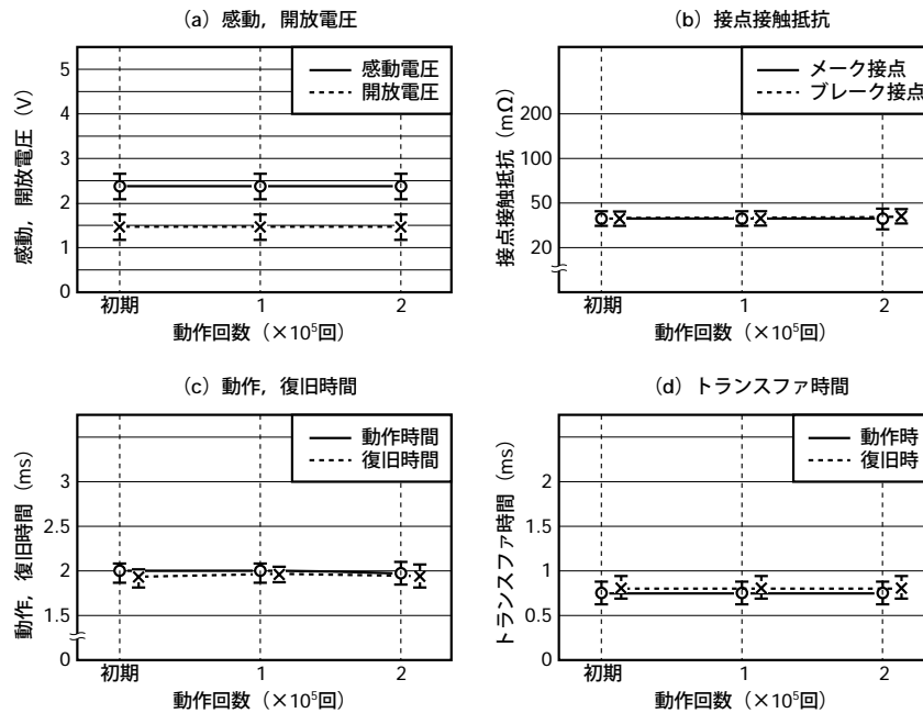
図5.19 抵抗負荷試験G
