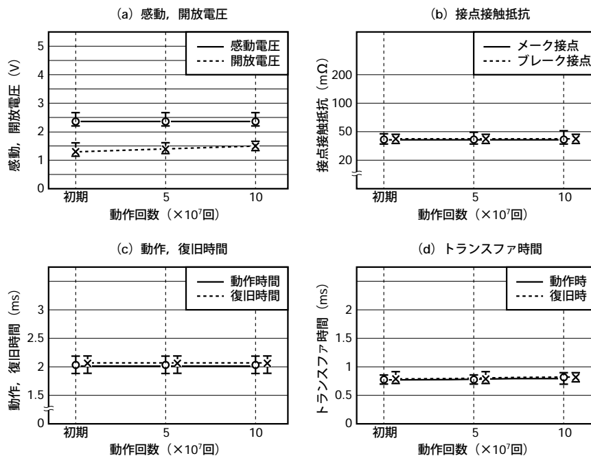
図5.10 無負荷試験A
