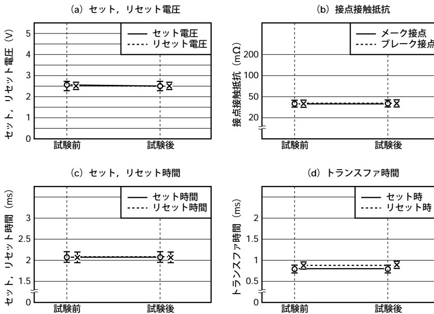
図5.5 (2) 振動
