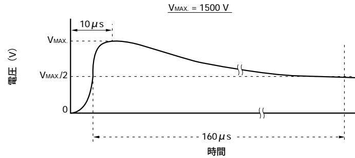
図3. 10 電圧サージ耐量
