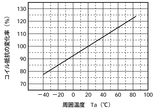
図3.7 温度特性
