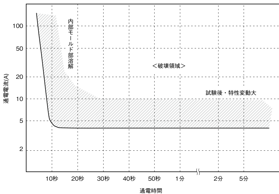
図3.12 通電耐量
