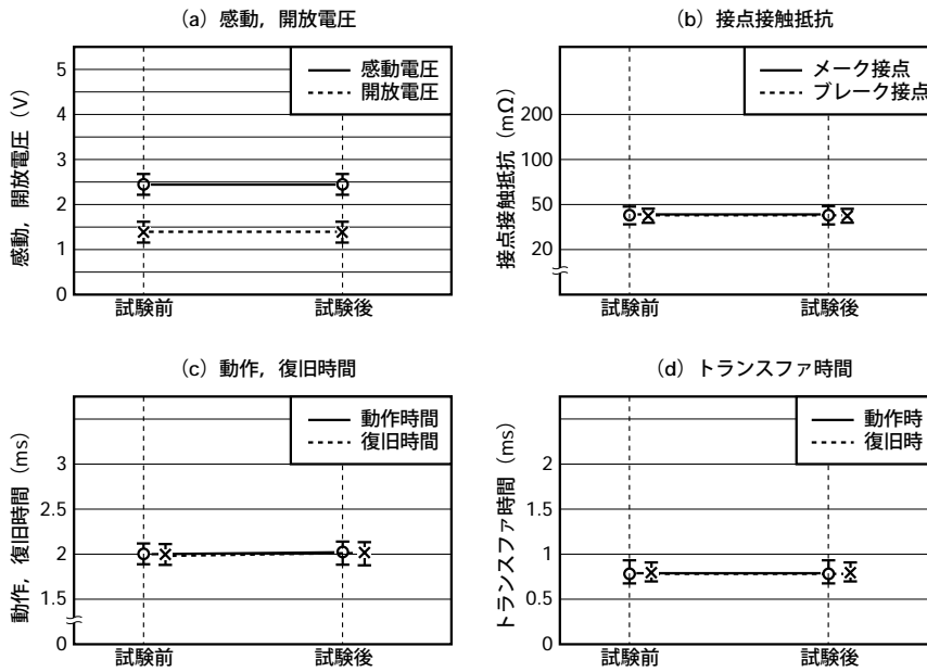
図5.7 (1) はんだ耐熱
