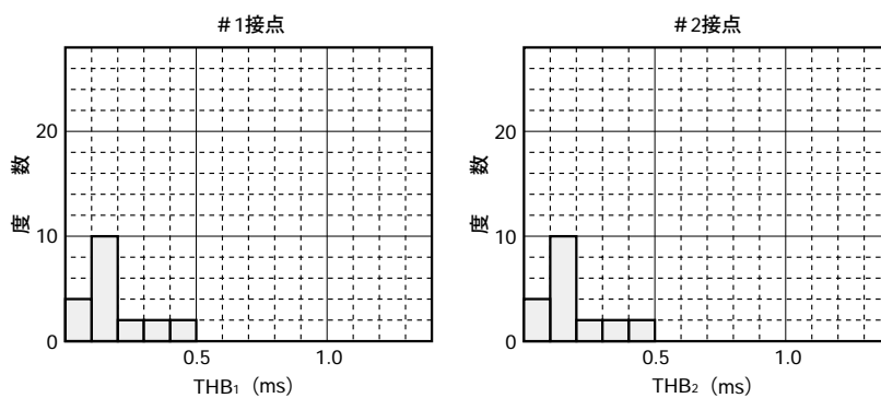
図4.4C 時間特性
