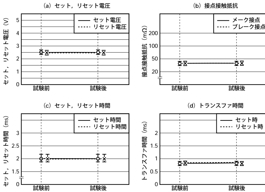
図5.2 (2) 低温放置
