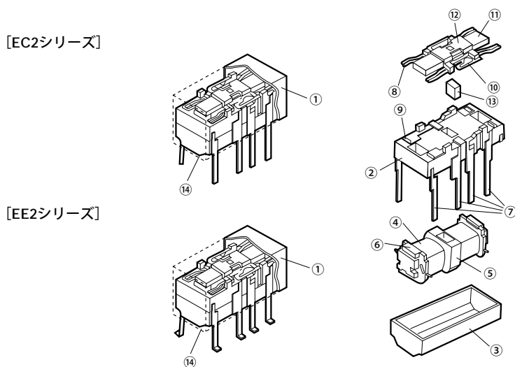
図2.1 EC2/EE2シリーズの構造
