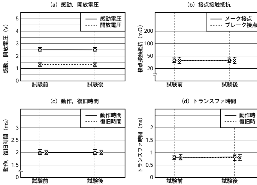
図5.1 (3) 高温放置
