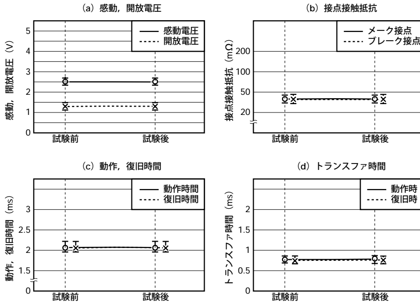
図5.2 (1) 低温放置
