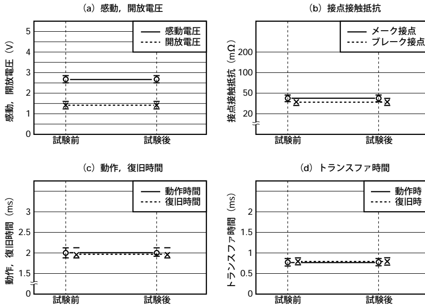
図5.3 (3) 温湿度サイクル
