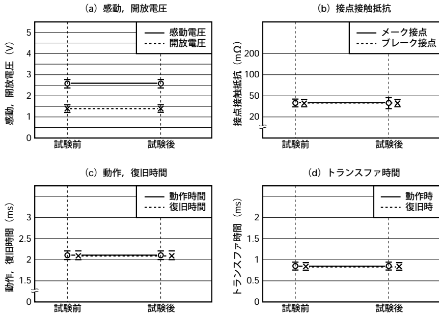
図5.5 (3) 振動
