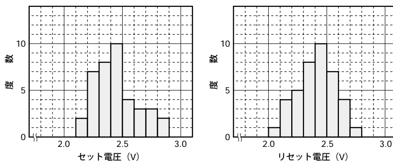
図4.1 感動・開放電圧
