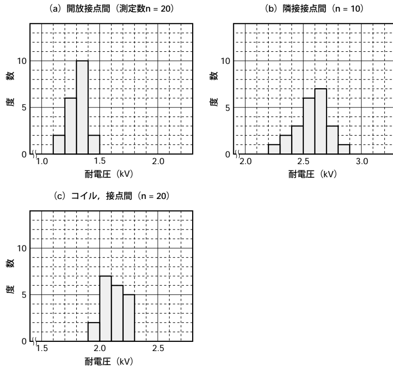
図4.6 耐電圧
