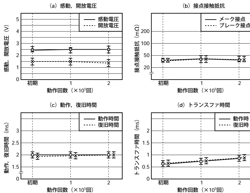
図5.20 抵抗負荷試験H
