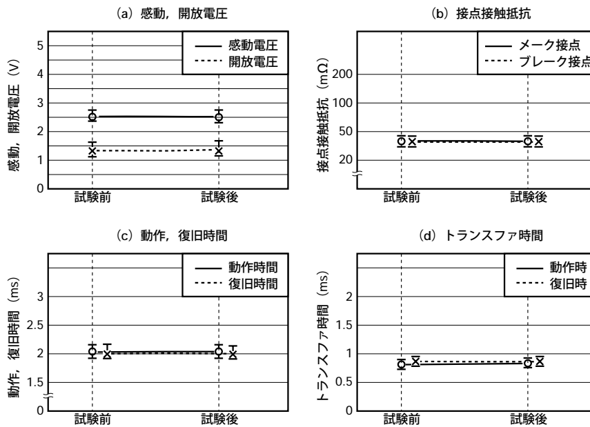
図5.1 (1) 高温放置
