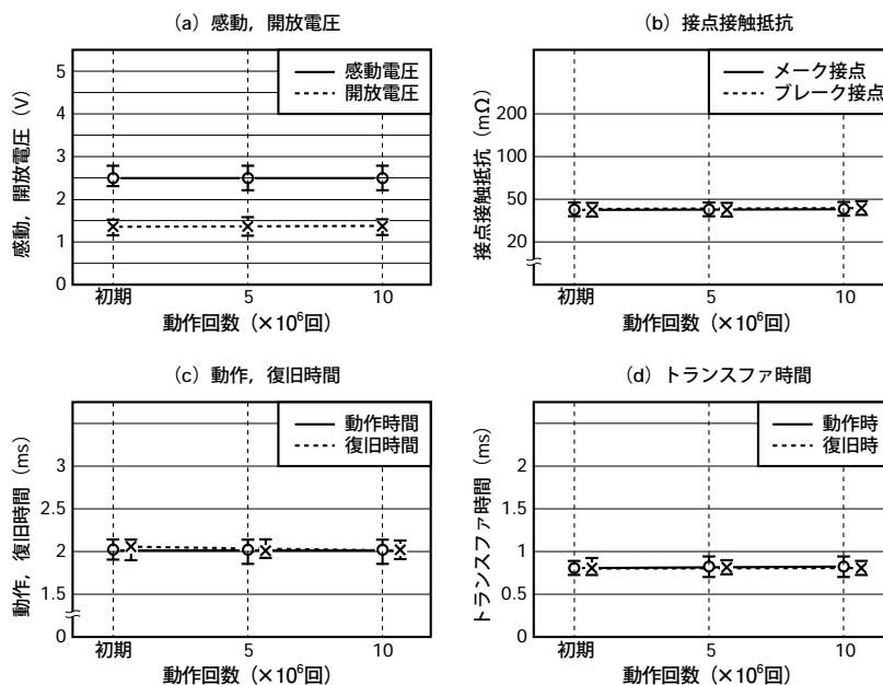
図5.12 抵抗負荷試験A
