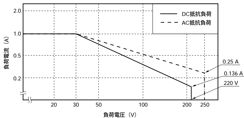
図3. 1 開閉容量
