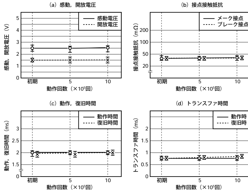
図5.13 抵抗負荷試験B
