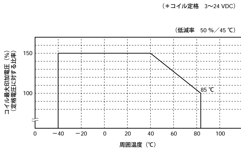
図3.3 コイル最大印加電圧
