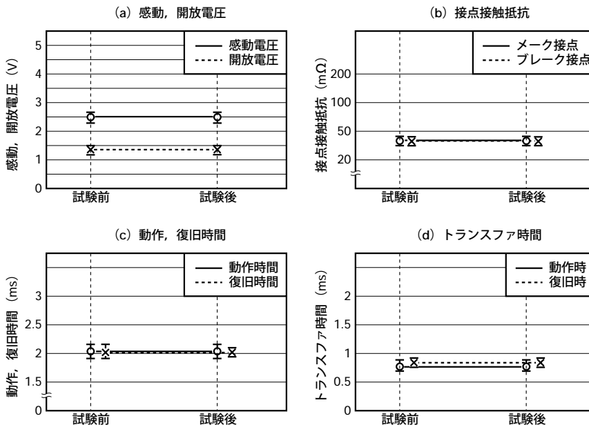
図5.5 (1) 振動
