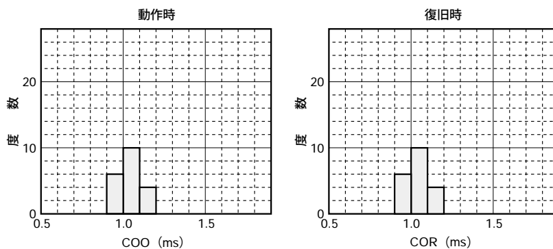
図4.4D 時間特性
