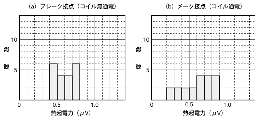
図4.7 熱起電力
