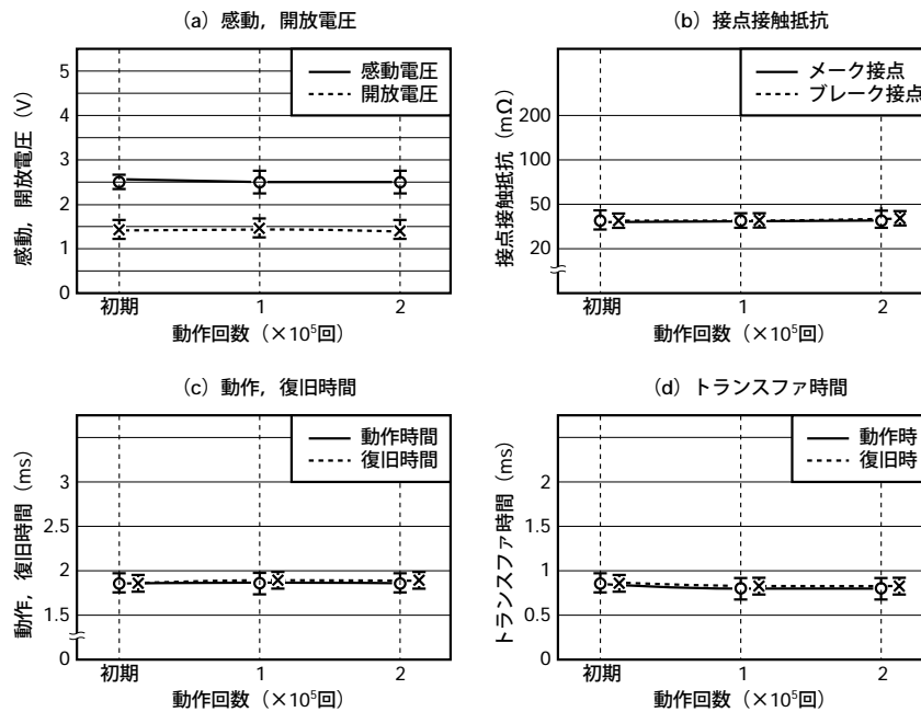
図5.18 抵抗負荷試験F
