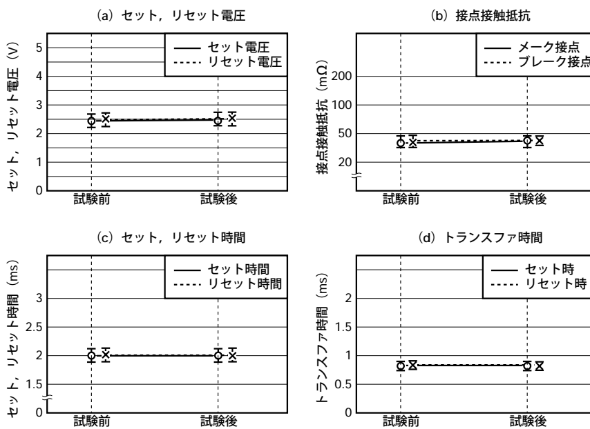
図5.7 (2) はんだ耐熱
