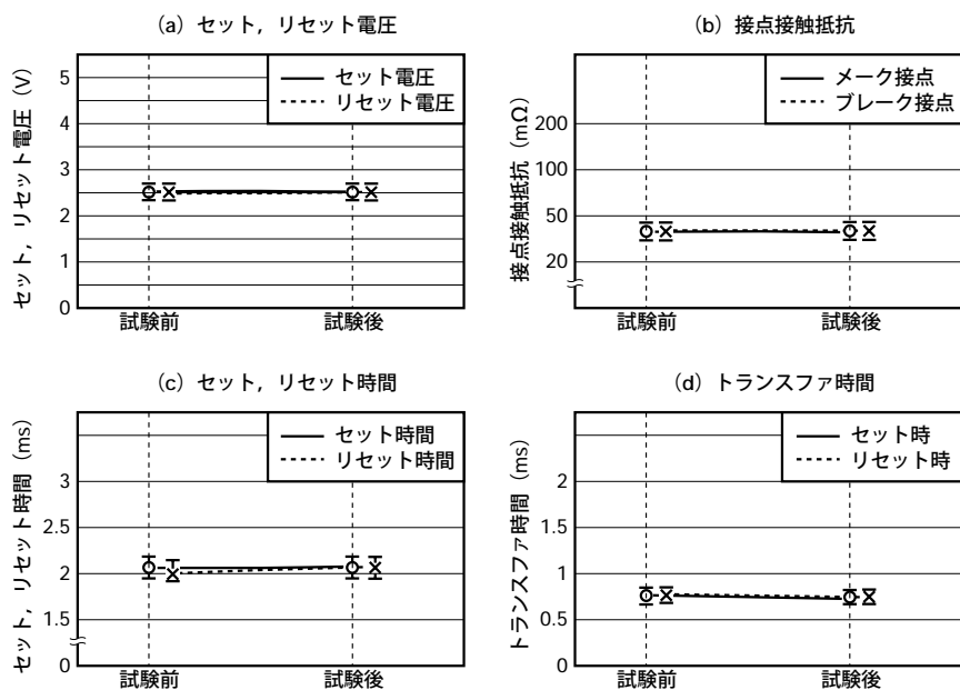
図5.1 (2) 高温放置
