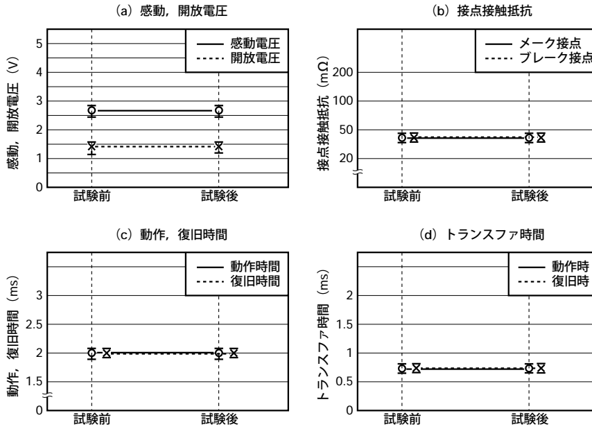
図5.4 (1) 熱衝撃
