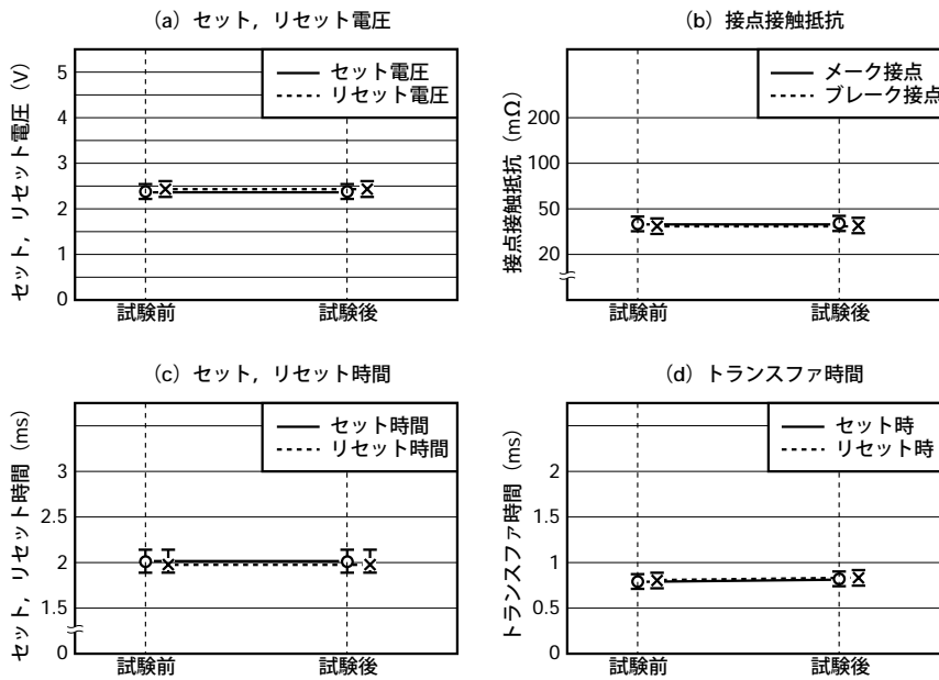
図5.4 (2) 熱衝撃
