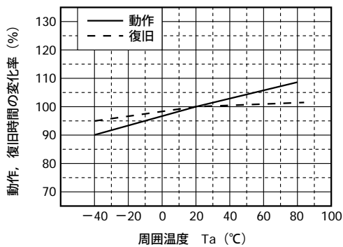
図3.7 温度特性
