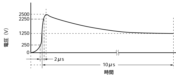
図3. 11 電圧サージ耐量
