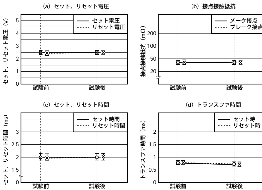
図5.9 (2) 端子強度
