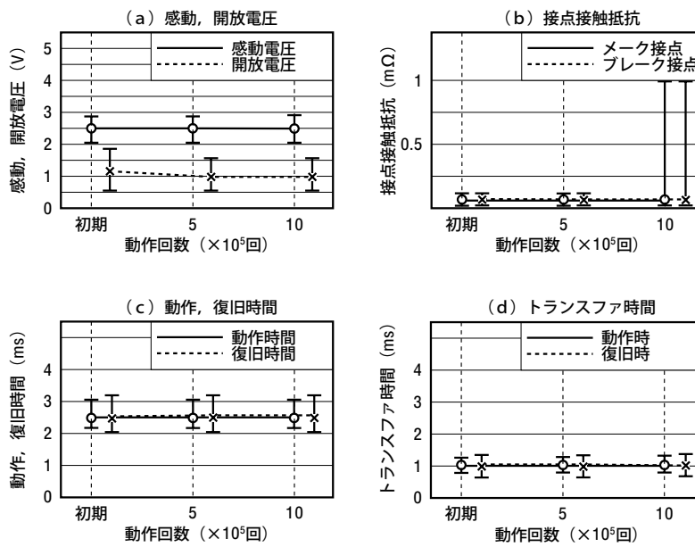
図5-11 抵抗負荷試験A
