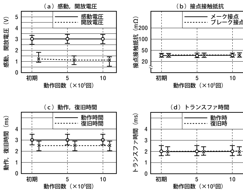
図5-12 抵抗負荷試験B
