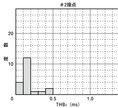
図4-4 (C) 時間特性
