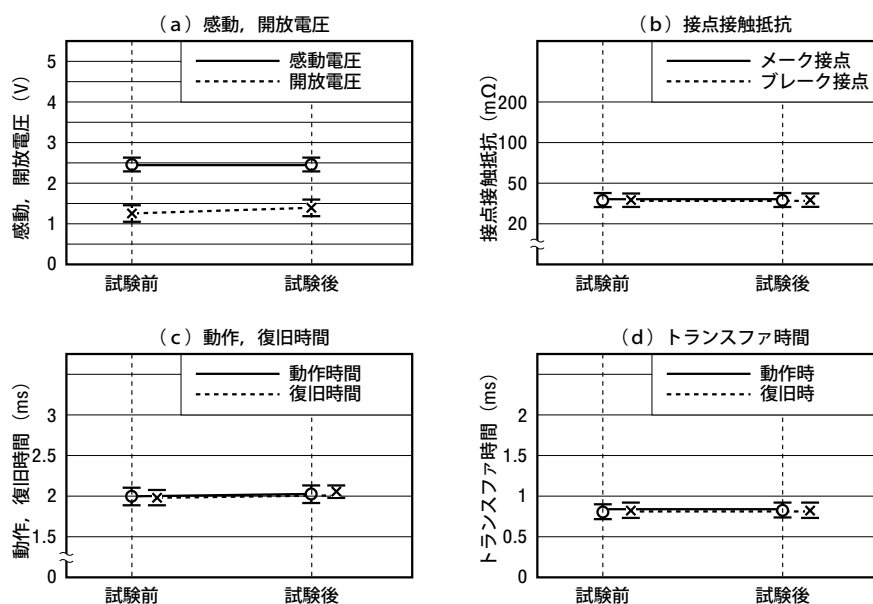
図5-9 端子強度
