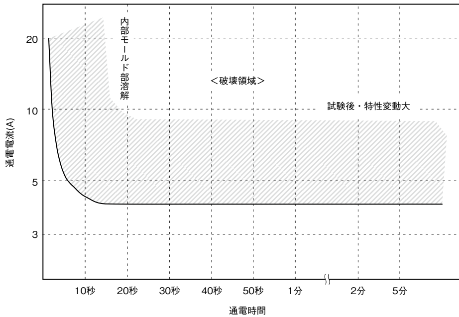
図3-10 通電耐量
