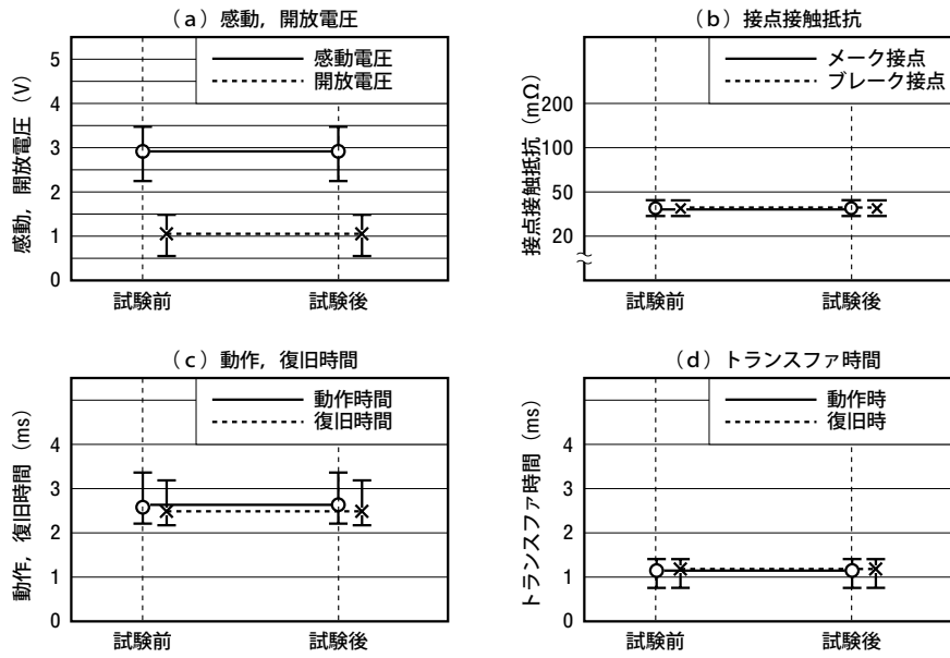
図5-4 熱衝撃
