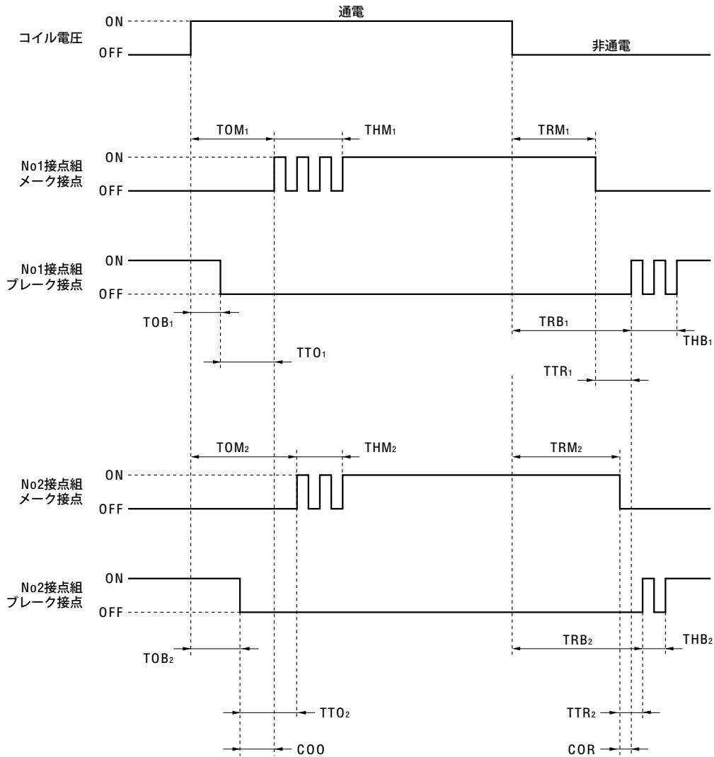
図4-4 (A) コイル, 接点のタイミングチャート
