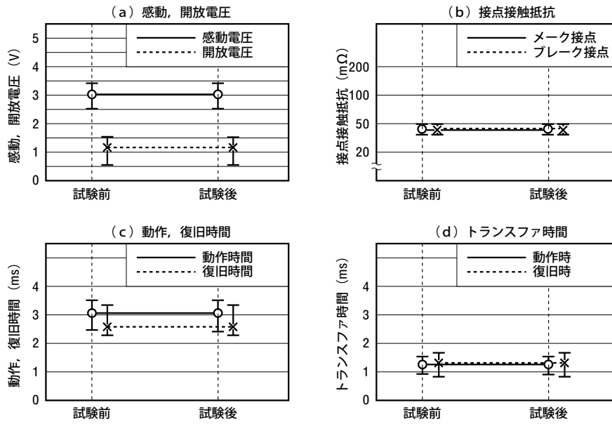
図5-2 低温放置
