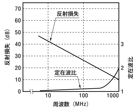
図3-7 高周波特性
