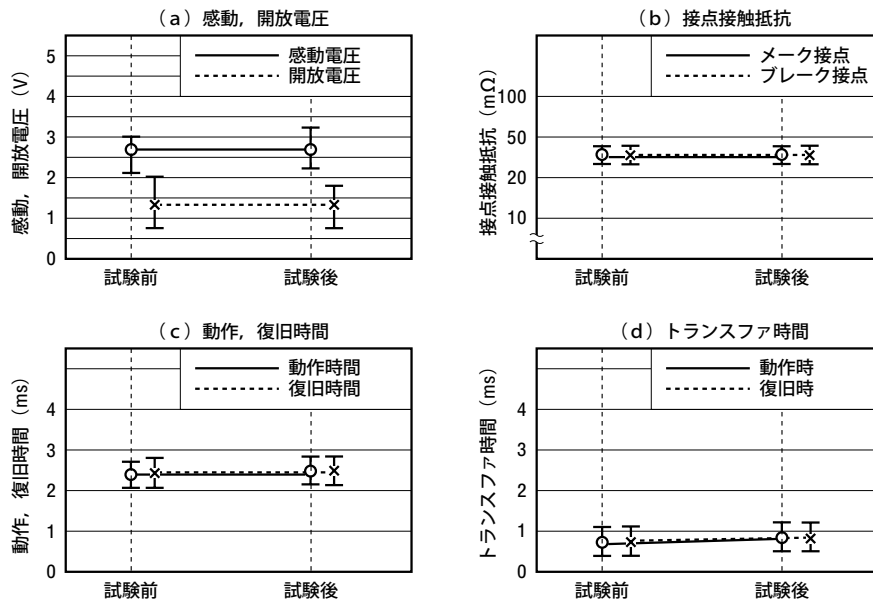
図5-8(2) リフローはんだ耐熱
