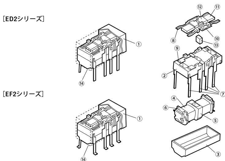
図 2-1 ED2/EF2シリーズの構造
