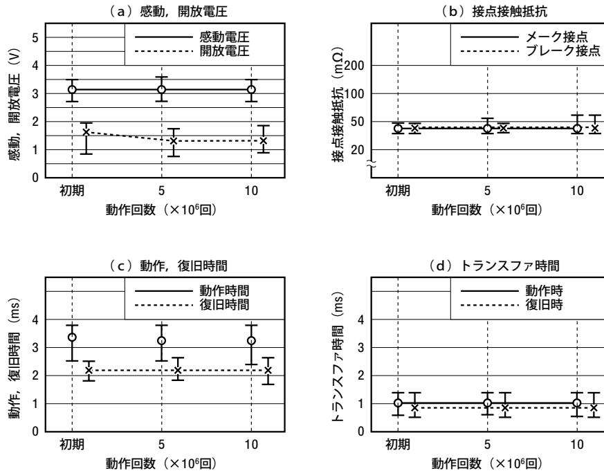
図5-10 無負荷試験
