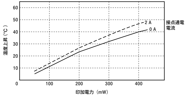
図3-3 コイル温度上昇
