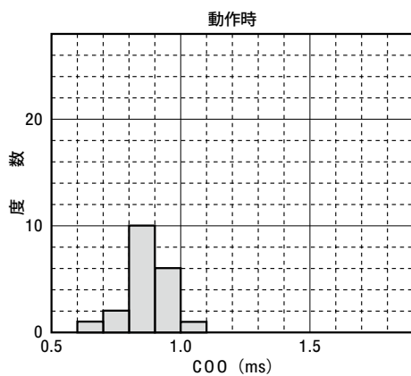
図4-4 (D) 時間特性
