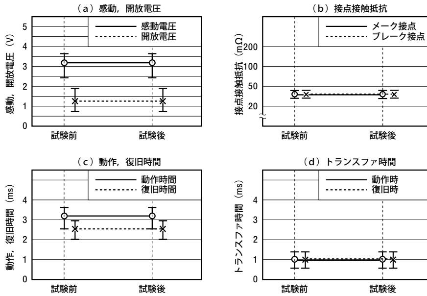
図5-6 衝撃
