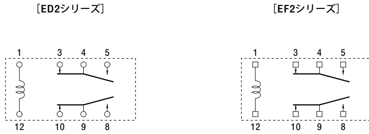
リレーの内部接続 (リレー底部より見て)
