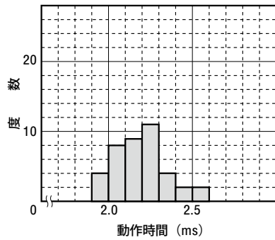
図4-2 動作, 復旧時間
