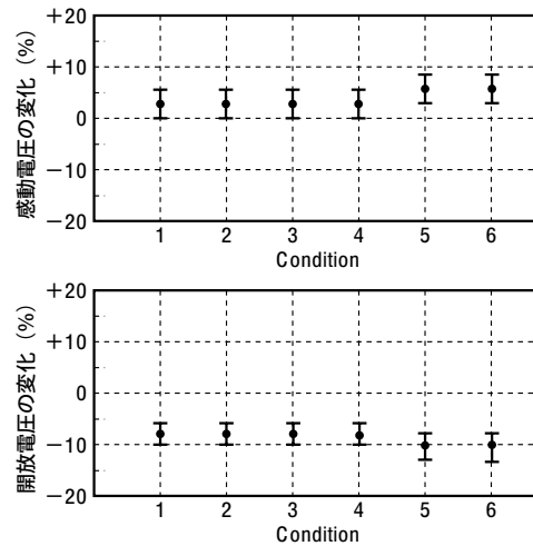
図3-6 磁気干渉
