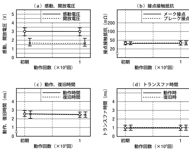
図 5-13 抵抗負荷試験C
