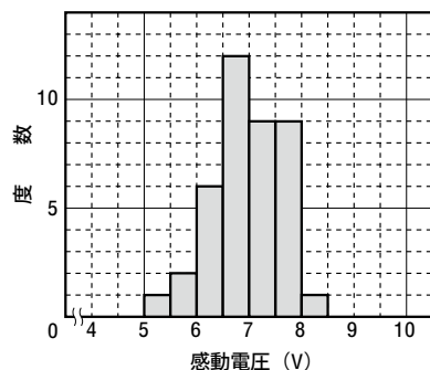
図4-1 感動・開放電圧
