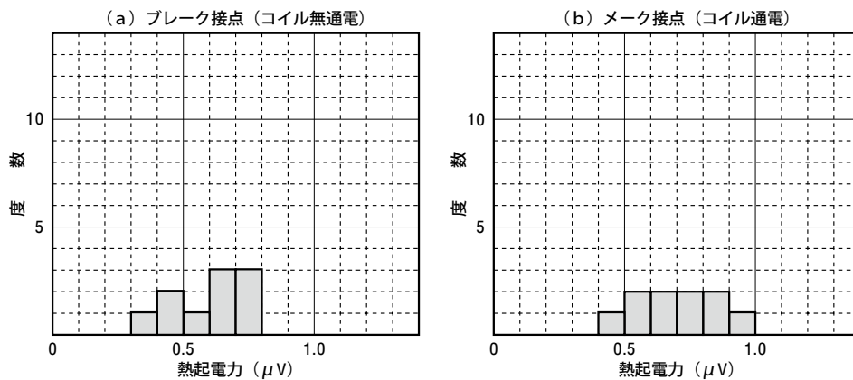
図4-7 熱起電力
