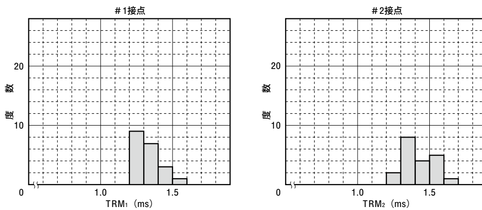
図4-4 (B) 時間特性
