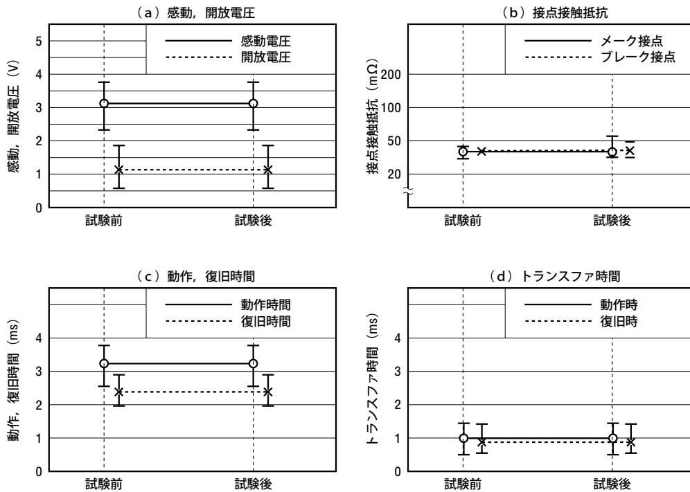
図 5-1 高温放置
