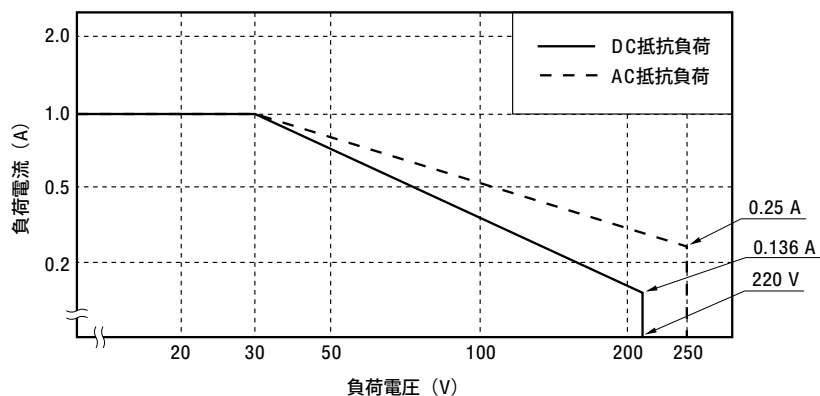
図3-1 開閉容量
