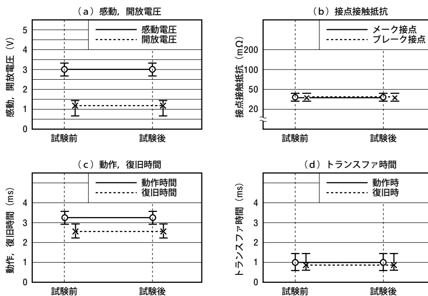
図5-5 振動
