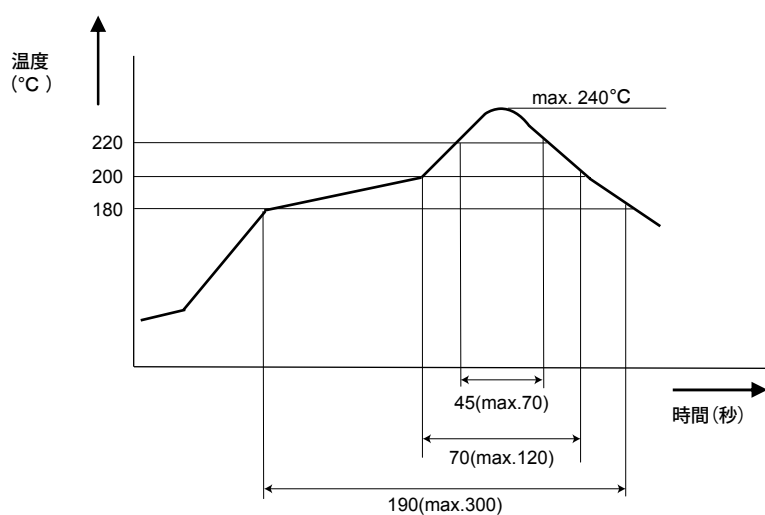
図5-8(1) 温度プロファイル
