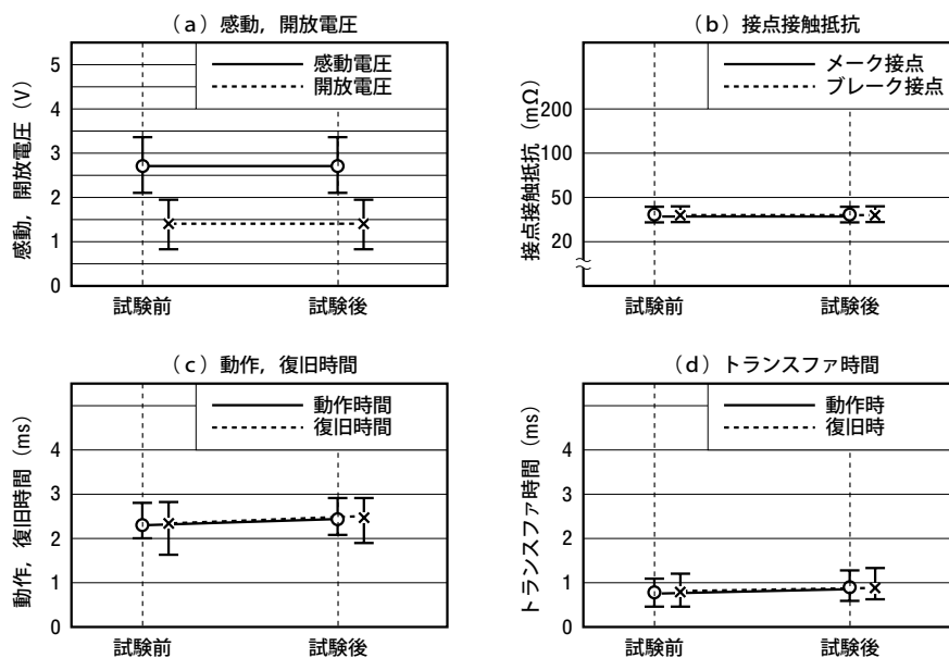
図5-7 はんだ耐熱
