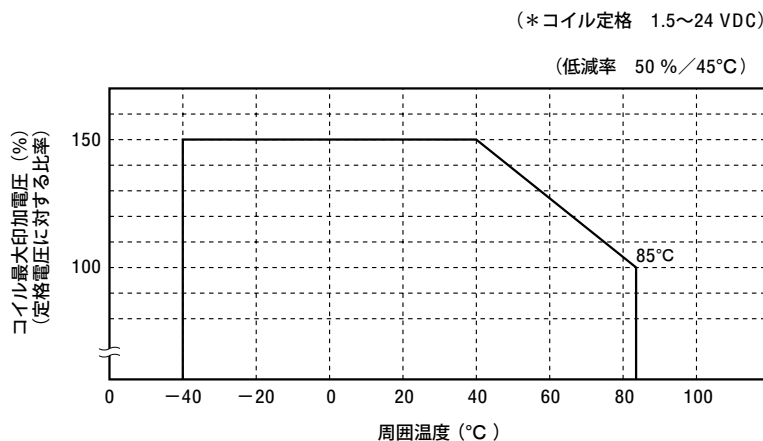
図3-2 コイル最大印加電圧
