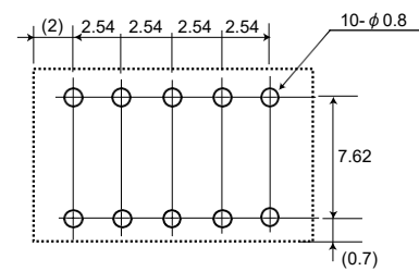
プリント配線板推奨実装パッド (Bottom view)
