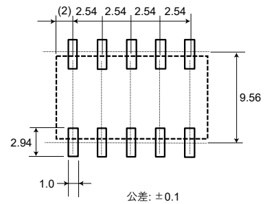
プリント配線板推奨実装パッド (Top view)
