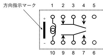
ノンラッチング型
