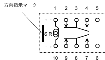
1巻線ラッチング型
