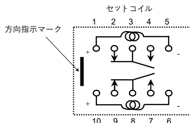
2巻線ラッチング型
