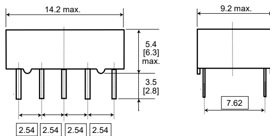
外形寸法
