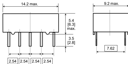
外形寸法
